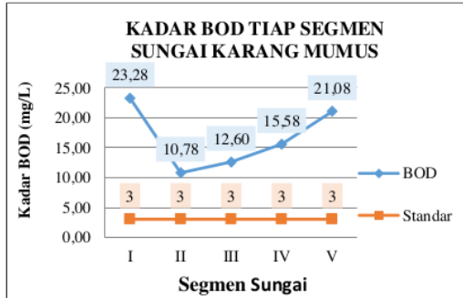
Gambar 2. Grafik Kadar BOD Tiap Segment Sungai Karang Mumus
