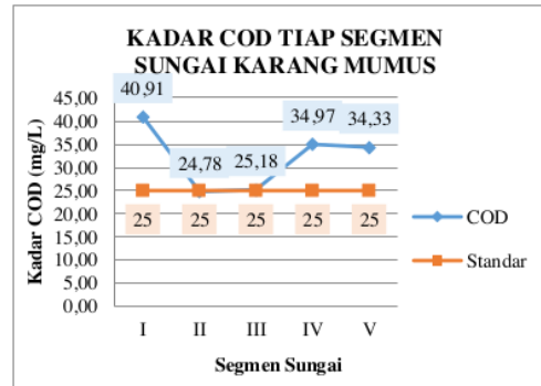
Gambar 3. Grafik Kadar COD Tiap Segment Sungai Karang Mumus
