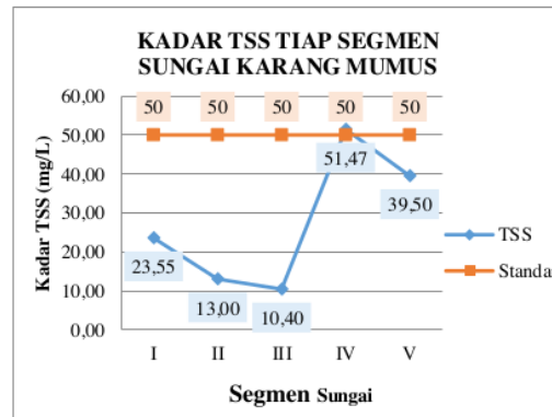
Gambar 4. Grafik Kadar TSS Tiap Segment Sungai Karang Mumus
