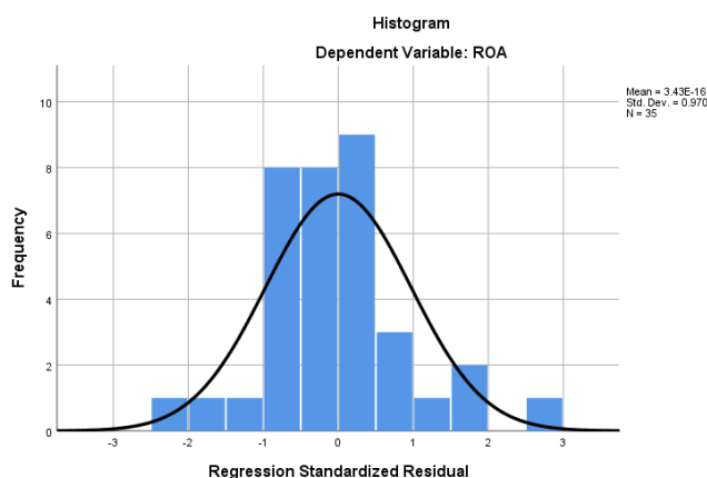
Gambar 2 : Grafik Histogram
