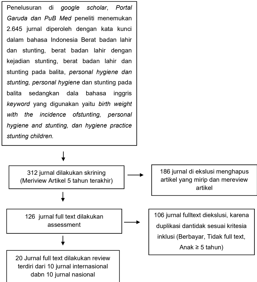
Gambar 3.2 Seleksi Studi dan Penelitian Kualitas
