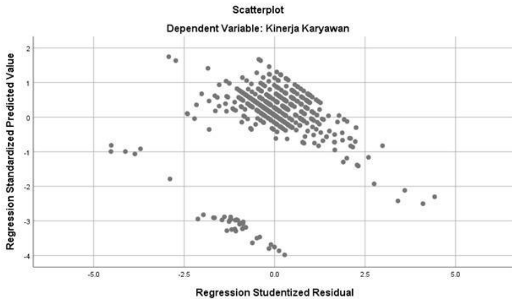
Gambar 2. Uji Heteroskedastisitas
