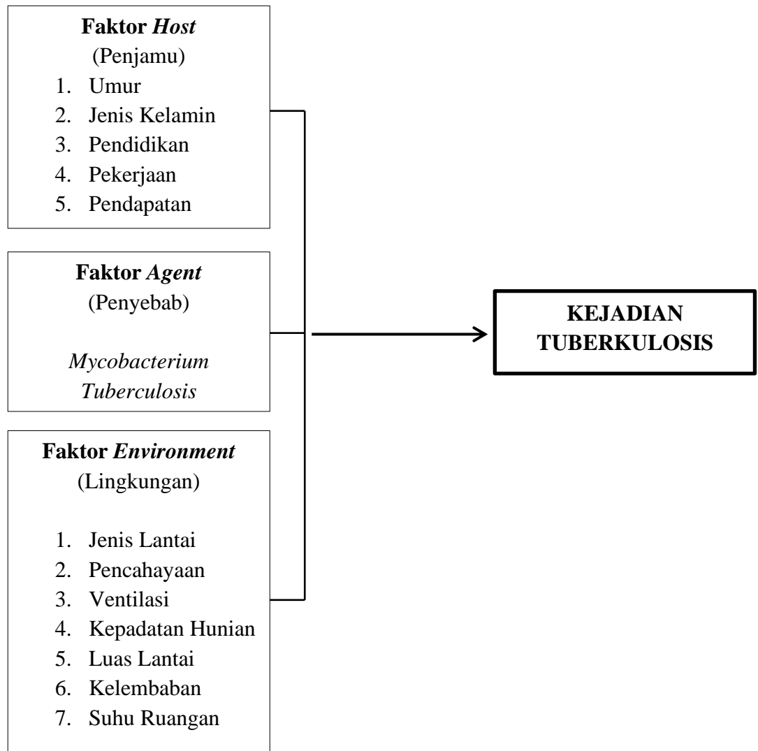
Gambar 1.2 Kerangka Teori
