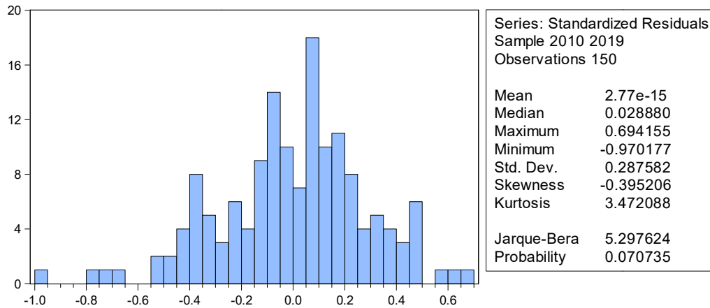
Gambar 2 Uji Normalitas
