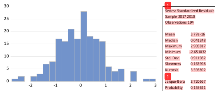
Gambar 2 Histogram dengan Data Tranformasi Log
