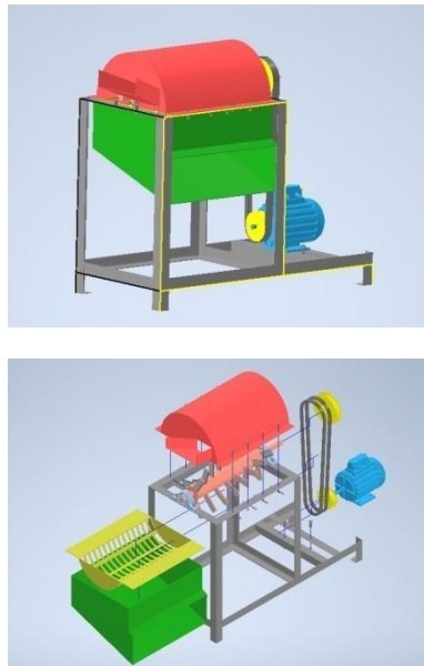
Gambar 1. Mesin Pencacah
