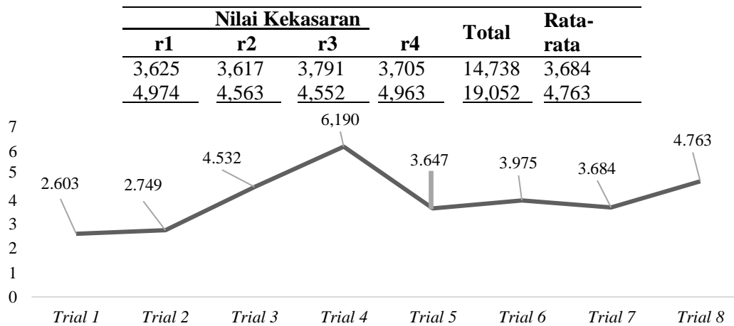
Gambar 1. Grafik nilai rata-rata kekasaran hasil pembubutan
