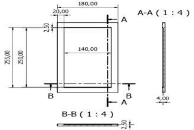
Gambar 3. Desain dan ukuran cetakan
