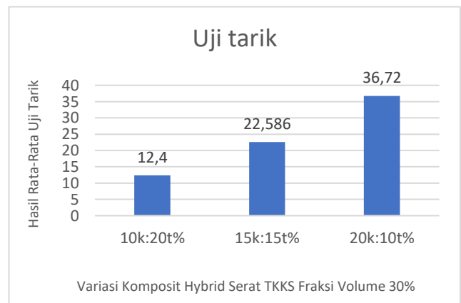
Gambar 8. Grafik kekuatan tarik rata-rata komposit hybrid
