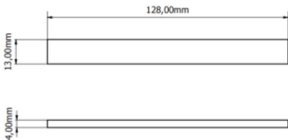
Gambar 5. Dimensi Spesimen Uji Bending (ASTM D7264)
