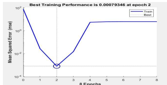
Gambar 3.1 Nilai Error
