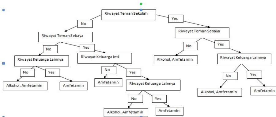
Gambar 1. Decision Tree dengan Algoritma C4.5.
