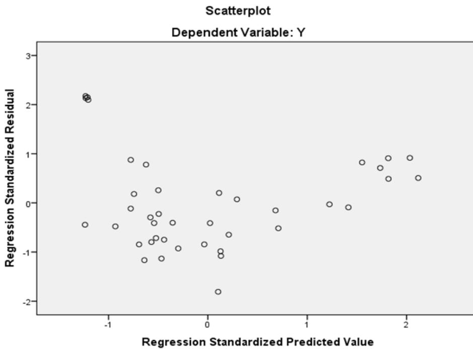
Gambar 1 Uji Heteroskedastisitas
